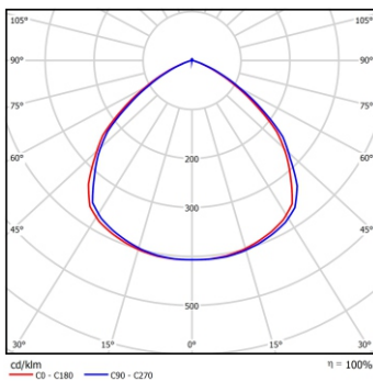
ToLEDo High Bay 100W con Cubierta
